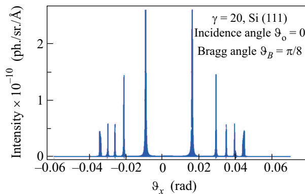
Рис. 5. Зависимость углового распределения DCR от угла \vartheta_x (при \vartheta_y = 0 ) для электронов с \gamma = 20 , падающих на плоскость (111) Si под углом \vartheta_0 = 0 ; наблюдение ведется под углом 2\vartheta_B = \pi/4
