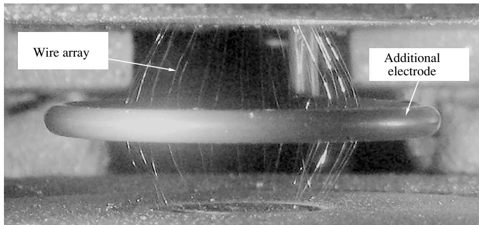
Рис.1. Фотография многопроволочного квазисферического лайнера в концентраторе тока установки Ангара-5-1. Зазор между основными электродами 15 мм, катод внизу, 40 вольфрамовых проволок диаметром 6 мкм длиной 17 мм. Дополнительный тороидальный электрод: малый диаметр 2.4 – мм, большой диаметр – 27.2 мм
