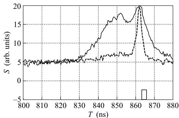
Рис.3. Рентгеновские сигналы S с датчиков ВРД1 и ВРД4. ВРД1 – сплошная линия, ВРД4 – пунктир. Нагрузка лайнера из 40 вольфрамовых проволок диаметром 6 мкм. Амплитуда тока 3 МА. Амплитуда напряжения между основными электродами концентратора тока в месте расположения дополнительного электрода 500 кВ. Прямоугольник соответствует моменту экспозиции всех кадров на рис.4
