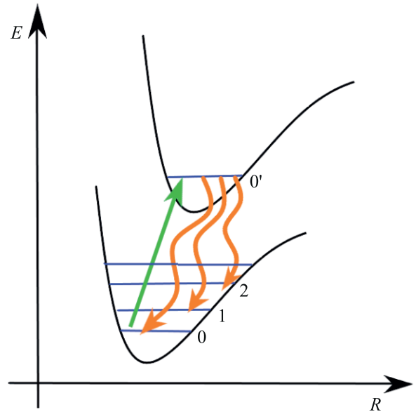
Рис. 1. (Цветной онлайн) Схема колебательных уровней для некоторой модельной двухатомной молекулы. Межъядерное расстояние ( R ) и энергия ( E ) даны в произвольных единицах. Цифры (0, 1, 2...) нумеруют колебательные уровни, штрих означает, что колебательный уровень принадлежит возбужденному электронному состоянию
