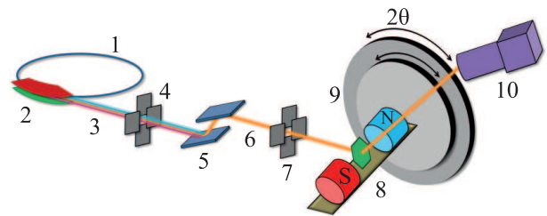
Рис. 1. (Цветной онлайн) Принципиальная схема дифракционного эксперимента. Здесь: 1 – накопительное кольцо источника синхротронного излучения; 2 – поворотный магнит, 3 – “белый” синхротронный пучок; 4 – входная маска (щель) “белого” пучка; 5 – двухкристальный монохроматор Si 111; 6 – монохроматичный рентгеновский пучок с энергией 12 кэВ; 7 – рентгеновские щели; 8 – экспериментальная ячейка с исследуемым кристаллом и электромагнитами (см. ниже); 9 – многокружковый гониометр; 10 – двумерный детектор
