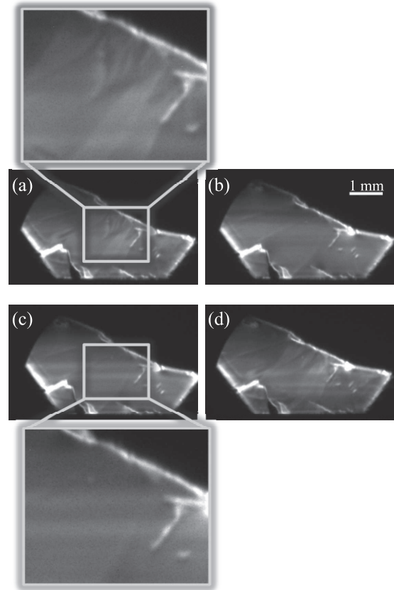
Рис. 4. Рентгеновские топограммы монокристалла \text{Fe}_{0.94}\text{Ga}_{0.06}\text{VO}_3 , полученные для рефлекса 300 без приложения внешнего магнитного поля (a), во внешнем магнитном поле 14 Э (d) и 40 Э (c), а также после отключения внешнего магнитного поля (d). На вставках показаны увеличенные фрагменты топограмм
