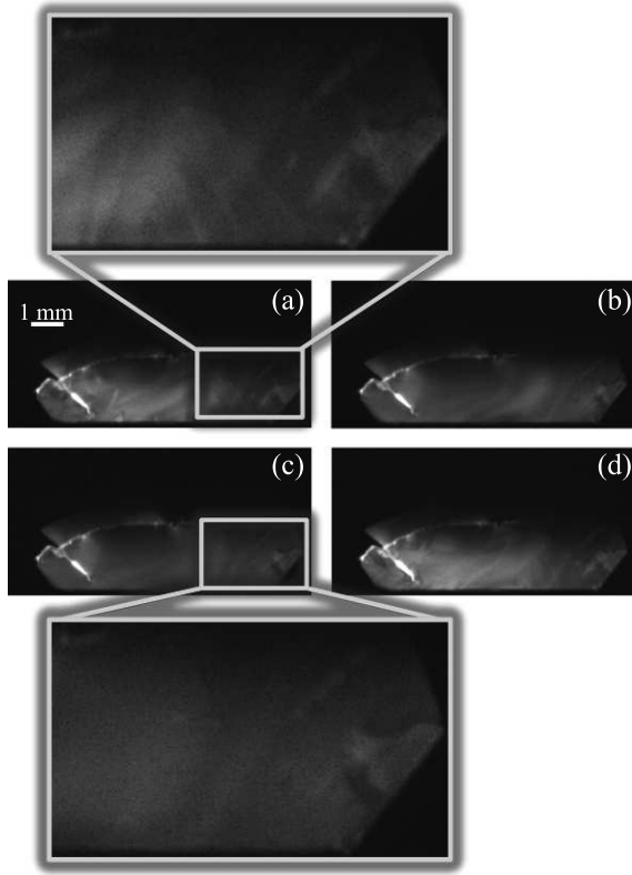
Рис. 3. Рентгеновские топограммы монокристалла \text{FeVO}_3 , полученные для рефлекса 300 без приложения внешнего магнитного поля (a), во внешнем магнитном поле 14 Э (b) и 40 Э (c), а также после отключения внешнего магнитного поля (d). На выносках показаны увеличенные фрагменты топограмм
