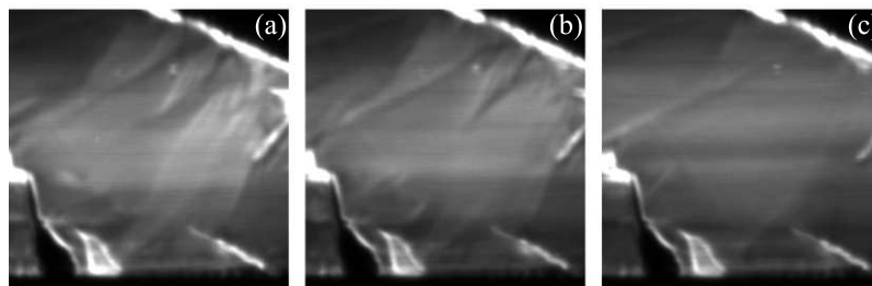
Рис. 6. Рентгеновские топограммы монокристалла \text{Fe}_{0.94}\text{Ga}_{0.06}\text{VO}_3 , полученные для рефлекса 300 без приложения внешнего магнитного поля (а), во внешнем магнитном поле \sim 1 Т (b) и \sim 2 Т (c)
