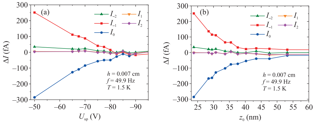
Рис. 4. (Цветной онлайн) (а) – Амплитуда изменения токов на сегментах коллектора при изменении прижимающего напряжения. (б) – Амплитуда изменения токов как функция глубины расположения квазидвумерного заряженного слоя. Температура T = 1.5 K
