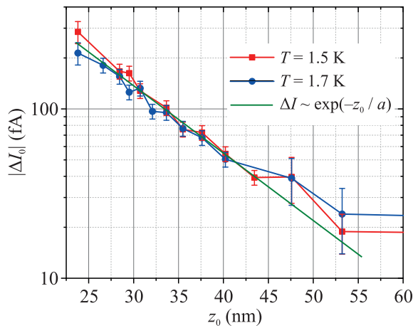
Рис. 5. (Цветной онлайн) Отклонение токов |\Delta I_0| на центральном сегменте коллектора при изменении расстояния от квазидвумерного заряженного слоя до поверхности жидкого гелия z_0 . Аппроксимирующая функция \sim \exp(-z_0/a) представлена зеленой прямой. Температуры измерений T = 1.5 и 1.7 K
