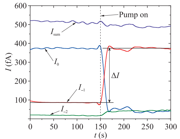
Рис. 2. (Цветной онлайн) Зависимость от времени токов отрицательных зарядов, приходящих на центральный “0”-ой сегмент I_0 , на “–1”-й сегмент I_{-1} и на “–2”-ой сегмент I_{-2} , I_{\text{sum}} – суммарный ток. Накачка волн плунжерами включается при t = 150 \text{ с} и выключается при t = 300 \text{ с} . Температура T = 1.5 \text{ К} , амплитуда волн накачки h = 0.007 \text{ см}
