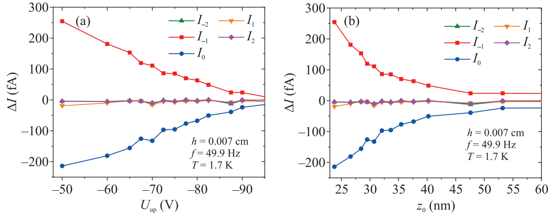
Рис. 3. (Цветной онлайн) (а) – Амплитуда изменения токов на сегментах коллектора при изменении прижимающего напряжения. (б) – Амплитуда изменения токов как функция глубины расположения квазидвумерного заряженного слоя. Температура T = 1.7 K
