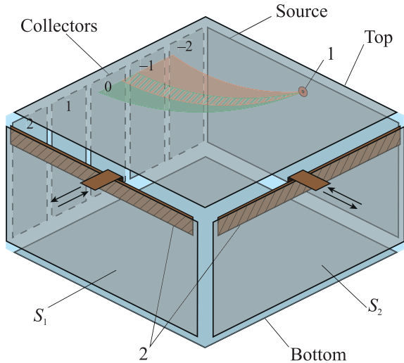
Рис. 1. (Цветной онлайн) Схема экспериментальной ячейки. 1 – источник зарядов; 2 – плунжеры, стрелки рядом указывают направление движения плунжеров. Грань, на которой располагается источник, называется Source . Показаны верхняя грань Top и нижняя Bottom , а также боковые грани, параллельно которым располагаются плунжеры, S_1 и S_2 , и грань с 5-ю сегментами коллектора Collectors . Схематично показаны каналы движения отрицательных зарядов в отсутствии накачки (зеленый) и при накачке волн (оранжевый)
