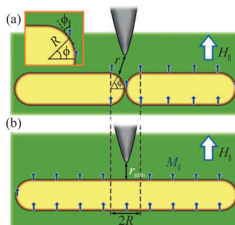
Рис. 5. (Цветной онлайн) Геометрия задачи: в теоретической модели головки расщепленных доменов представляются полуокружностями с радиусом R . Синими стрелками M_{\parallel} показана намагниченность внутри доменных границ. (a) – Положение участка стенки задается его расстоянием до источника поля r и углом \phi ; (b) – положение участка стенки в рассматриваемой области шириной 2R задается линейной координатой вдоль прямых участков стенки, r_{\min} – минимальное расстояние от электрода до доменной границы
