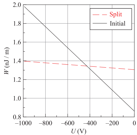
Рис. 6. (Цветной онлайн) Поверхностные энергии, проинтегрированные по длине участков, ближайших к игле (между вертикальными штриховыми линиями на рис. 5), для двух конфигураций: первоначального состояния полосового домена (initial) и расщепленного (split)
