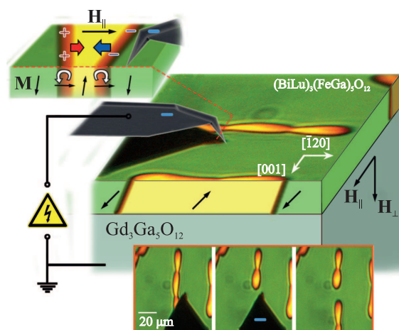
Рис. 3. (Цветной онлайн) Эффект расщепления доменов с перетяжкой. На вставках внизу: экспериментальные магнитооптические изображения до, во время и после электрического воздействия иглой. На вставке вверху: сечение перетяжки. Черными стрелками показано направление намагниченности и магнитных полей, белыми стрелками – кристаллографические направления, белыми круглыми стрелками – направление разворота намагниченности
