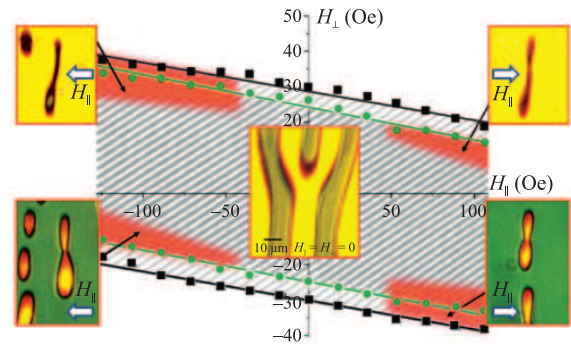
Рис. 2. (Цветной онлайн) Фазовая диаграмма в осях поле в плоскости пленки H_{\parallel} и поле перпендикулярно плоскости пленки H_{\perp} . Незаштрихованные части диаграммы – области монодоменных состояний, более плотной штриховкой показаны области, в которых существуют домены независимо от предыстории, менее плотной штриховкой показаны области гистерезиса, в которых метастабильные домены сохраняются только при движении в сторону больших по модулю полей. Символы соответствуют экспериментально измеренным границам монодоменного состояния: черные квадраты – при увеличивающемся по модулю поле H_{\perp} , зеленые круги – при уменьшающемся; линии соответствуют аппроксимации линейной зависимости. Цветом выделены области фазовой диаграммы, соответствующие существованию доменов с перетяжками, в которых наблюдается эффект расщепления доменов. На вставках показаны магнитооптические изображения доменов с перетяжками, наблюдающиеся во всех четвертях диаграммы, и соответствующие им направления поля H_{\parallel}
