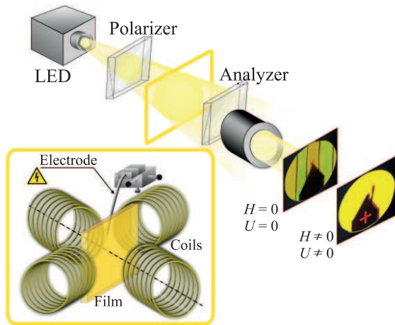
Рис. 1. (Цветной онлайн) Схема экспериментальной установки для визуализации доменной структуры и локального воздействия электрическим полем: подсветка осуществляется белым светодиодом (LED), исследуемый образец находится между поляризатором (polarizer) и анализатором (analyzer), скрещенными под углом, близким к \pi/2 . На вставках показаны магнитооптические изображения микромагнитной структуры и заостренный наконечник электрода (темный объект)
