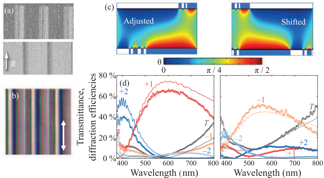
Рис. 6. (Цветной онлайн) Двусторонняя ЖК-метаповерхность периода P = 8 мкм и толщины d = 4 мкм. (a) – РЭМ-изображения фрагментов подложек, покрытых ориентирующими слоями полиимида, натертыми в направлении стрелки R с облученными ФИП суперпериодическими полосами в соответствии с оптимизированным дизайном. (b) – Изображение в оптическом микроскопе метаповерхности в свете, поляризованном вдоль полос (белая стрелка). (c) – Цветовые карты распределения полярного угла директора ЖК в пределах одного периода при точном совмещении подложек (слева) и при сдвиге на половину периода (справа). (d) – Спектры коэффициента пропускания и дифракционных эффективностей для совмещенной конфигурации (слева) и смещенной на половину периода (справа). Сплошными линиями показаны смоделированные, а точками – измеренные значения [43]
