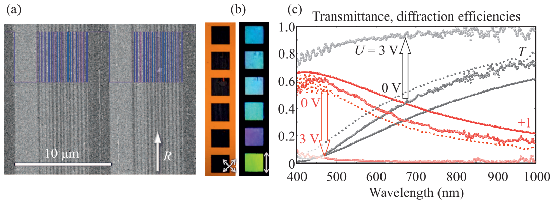
Рис. 5. (Цветной онлайн) Односторонние суперпериодические ЖК-метаповерхности. (а) – РЭМ-изображение фрагмента суперпериодической структуры периода P = 10 мкм, облученной ФИП. Ступенчатая зависимость полярного угла директора ЖК показана синей линией. (б) – Изображения в поляризационном оптическом микроскопе ЖК-ячейки с метаповерхностями P = 5\text{--}10 мкм (сверху вниз) и толщины d = 4 мкм, помещенной между парой скрещенных поляризаторов, повернутых на 45^\circ относительно полос (белые стрелки) и при наклонном падении света, линейно поляризованного вдоль полос. (с) Спектры коэффициента пропускания и дифракционных эффективностей структуры периода P = 10 мкм: сплошными линиями показаны результаты аналитической модели, пунктирными – численного моделирования, а точками – измеренные в отсутствие напряжения и при приложении напряжения [36]
