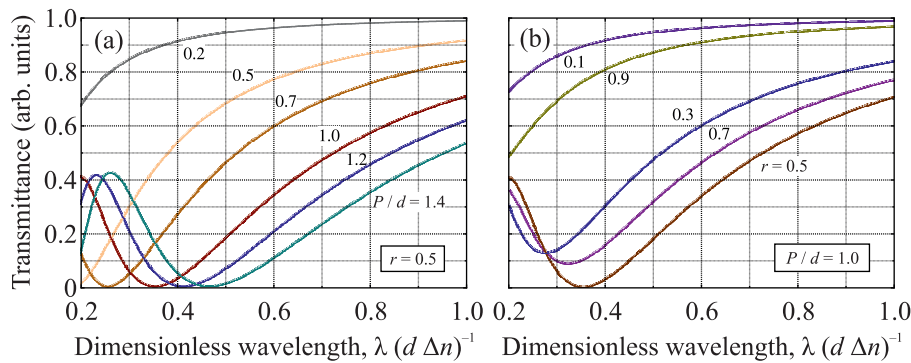
Рис. 2. (Цветной онлайн) Спектры коэффициента пропускания ЖК метаповерхностями нормально падающего света, поляризованного вдоль полос, рассчитанные по аналитическому выражению (3): для фиксированного значения коэффициента заполнения r = 0.5 и различных значений P/d (a), а также для фиксированного P = d и различных значений r (b) [33]
