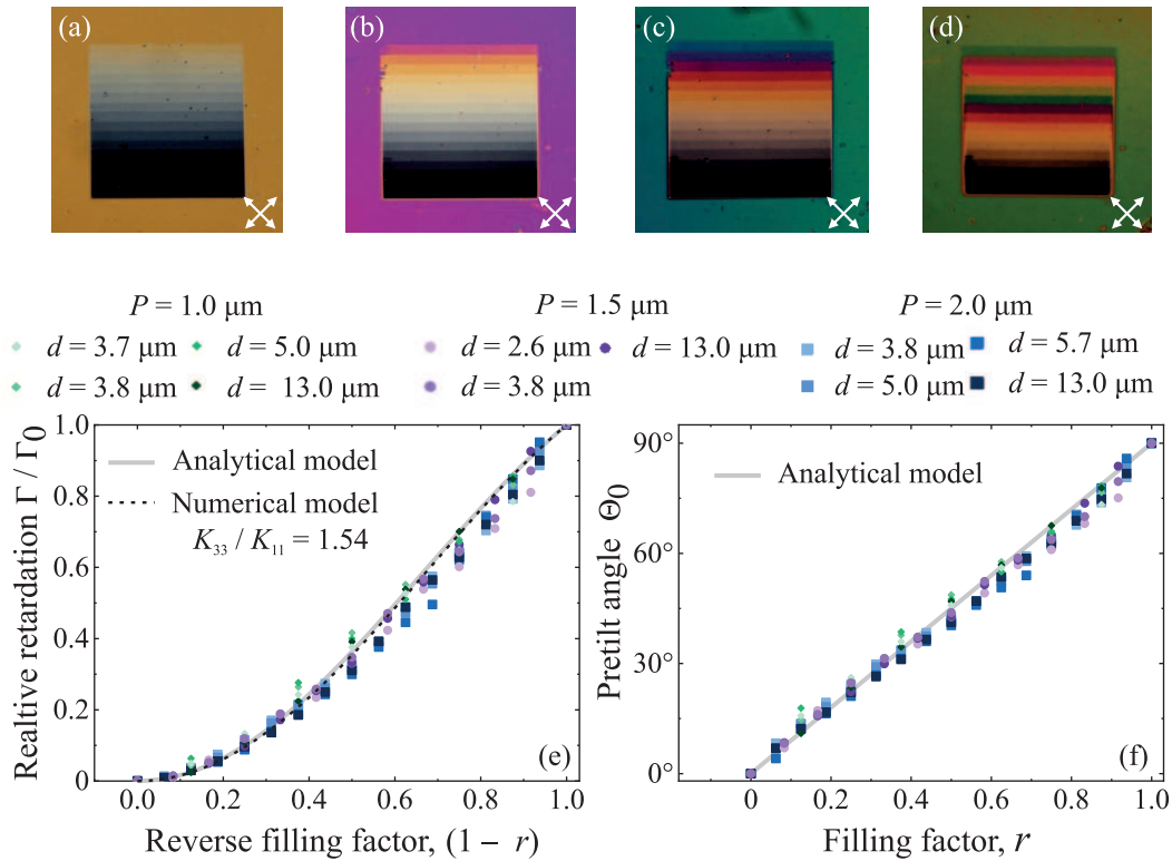
Рис. 4. (Цветной онлайн) Изображения в скрещенных поляризаторах (белые стрелки) ЖК-ячеек с метаповерхностями, формирующимися на периодических структурах с P = 2 мкм и коэффициентом заполнения, меняющимся от r = 0 на верхнем крае до r = 1 – на нижнем, для различных значений толщины слоя ЖК d : 3.8 мкм (а), 5.0 мкм (b), 6.5 мкм (с) и 13 мкм (d). Относительная фазовая задержка (е) и эффективный угол преднаклона (f) в зависимости от коэффициента заполнения, измеренные для ЖК-метаповерхностей с различными d и P (цветные символы) и рассчитанные по аналитическим формулам (6) и (8). Пунктирной линией на (е) также представлен результат расчета для модулей упругости нематика E7 [35]
