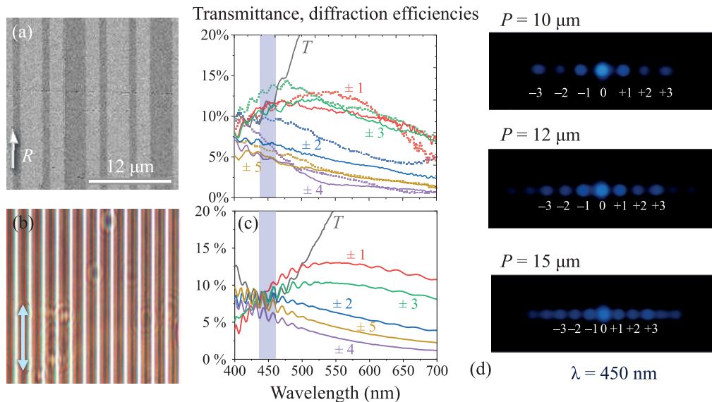
Рис. 7. (Цветной онлайн) Примеры ЖК-метаповерхностей – аналогов решеток Дамманна – толщины 4 мкм и различных периодов. (a) – РЭМ-изображение фрагмента структуры периода 12 мкм, записанной ФИП. Белой стрелкой R указано направление натирки полиимида. (b) – Изображение участка ЖК-метаповерхности в поляризационном оптическом микроскопе. Белой стрелкой указано направление поляризации света. (c) – Спектры пропускания и эффективностей первых 11 порядков дифракции этой же метаповерхности, измеренные в эксперименте (сверху) и смоделированные численно (снизу). (d) – Картины дифракции, зарегистрированные в задней фокальной плоскости оптического микроскопа для метаповерхностей указанных разных периодов [45]
