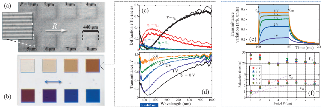
Рис. 3. (Цветной онлайн) Экспериментальный набор периодических ЖК-метаповерхностей периода от 1 до 8 мкм, сформировавшихся на полосах, обработанных ФИП с коэффициентом заполнения 0.5 [34]. РЭМ-изображения периодических полос, облученных ФИП с указанным периодом P (а). Белой стрелкой обозначено направление натирки полиимида R . Изображения ЖК-ячейки с плоским зазором толщиной d = 3.5 мкм, в котором сформировались метаповерхности, видимые в оптическом микроскопе в свете, линейно поляризованном вдоль полос (б). Спектры пропускания и эффективностей первых порядков дифракции (с), рассчитанные численно (сплошные линии) и измеренные (точки) для метаповерхности периода 4 мкм. Изменение спектра пропускания этой метаповерхности при приложении указанных напряжений 1–6 В (д). Динамика изменений коэффициента пропускания на длине волны 445 нм при приложении ступенчатых импульсов напряжения частотой 1.5 кГц указанной амплитуды (е). Времена быстрой (полые символы) и медленной (сплошные символы) релаксации метаповерхностей разного периода при различных напряжениях в сравнении с модельными зависимостями (5), показанными штриховыми линиями (ф)
