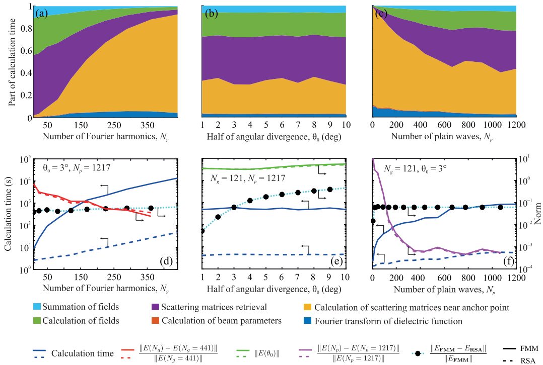
Рис. 3. (Цветной онлайн) (a)–(c) – Распределение общего времени расчета поля гауссова пучка, прошедшего через периодический слой, методом резонансного подпространства по вкладам от различных операций (показаны цветом на легенде снизу) в зависимости от числа фурье-гармоник N_g , от половины угла расходимости пучка \theta_0 и от числа плоских волн N_p . (d) – Зависимость времени расчета и точности вычисления поля гауссова пучка классическим ФММ и методом резонансного подпространства от указанных параметров
