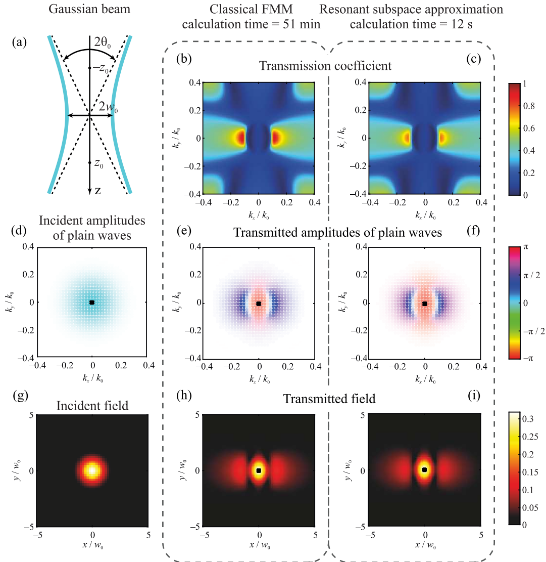
Рис. 2. (Цветной онлайн) (а) – Схема гауссова пучка. (d) – Комплексные амплитуды плоских волн, на которые разложен гауссов пучок с половиной угла расходимости \theta_0 = 8^\circ . (g) – Плотность энергии электрического поля пучка в сечении z = z_0 . (b) и (c) – Коэффициент пропускания |t_{yy}|^2 как функция компонент волнового вектора, рассчитанный при a/\lambda = 0.62 классическим ФММ и методом резонансного подпространства. (e) и (f) – Комплексные амплитуды распространяющихся плоских волн, прошедших через периодический слой. (h) и (i) – Плотность энергии электрического поля пучка, прошедшего через периодический слой, рассчитанная на расстоянии 10 мкм от нижней границы слоя классическим ФММ и методом резонансного подпространства. На панелях (d)–(f) модули комплексных амплитуд показаны яркостью точки (чем ярче, тем больше модуль), а аргументы (фазы) комплексных амплитуд – цветом; соответствие между цветом и фазой показано на цветовой шкале справа
