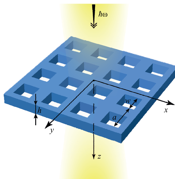
Рис. 1. (Цветной онлайн) Схема периодического слоя и нормально падающего на него гауссова пучка. Период структуры a = 1 мкм, ширина квадратных отверстий w = 0.6 мкм, толщина слоя h = 0.1 мкм
