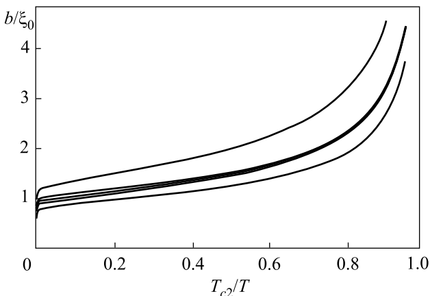
Рис.1. Зависимость относительной длины экстраполяции b/\xi_0 от относительной температуры перехода контактирующих сверхпроводников. Кривые сверху вниз: для одномерного сверхпроводника, для d_{xy} -, s -, d_{x^2-y^2} -двухмерных, для трехмерного
