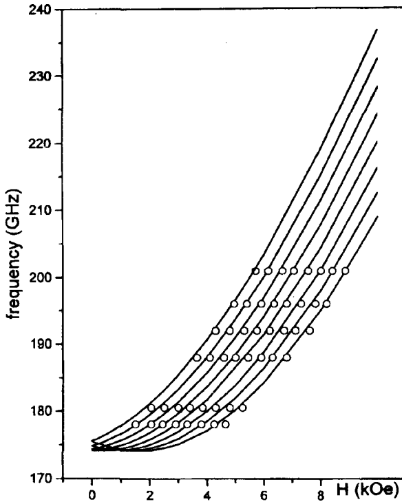
Рис.3. Вычисленные частоты магнитных дипольных переходов в кристалле KY_3F_{10}: Ho^{3+} при H \parallel H_1 \parallel C_4 . Результаты измерений представлены кружками
