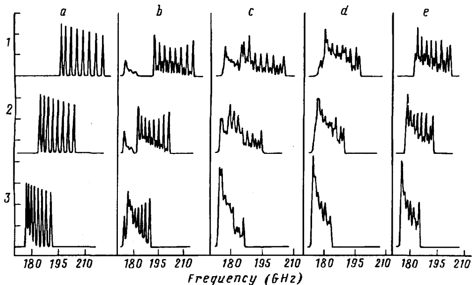
Рис.1. Вычисленные спектры поглощения кристалла \text{KY}_3\text{F}_{10}:\text{Ho}^{3+} в параллельных полях в зависимости от величины постоянного магнитного поля (1 - H=8 кЭ, 2 - H=6 кЭ, 3 - H=4 кЭ) и его ориентации в плоскости (1 1 0). Угол \varphi между H и кристаллографической осью [0 0 1] равен: a - 0°, b - 20°, c - 40°, d - 60°, e - 90°
